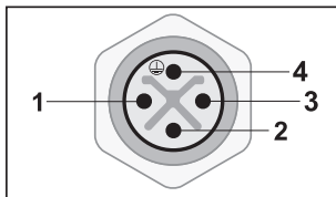
Schemazeichnung M12 S-kodiert
