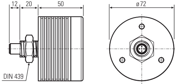
1 SPOTLED II Aufbau
