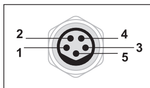
Schemazeichnung M8-Stecker
