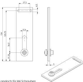
Langloch für M6 Schrauben Befestigungselemente Leuchtenseitig im Lieferumfang enthalten
