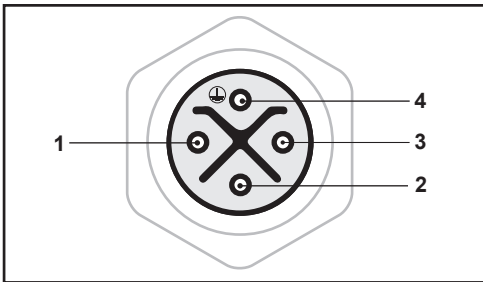
Schemazeichnung M12-Stecker, S-kodiert
