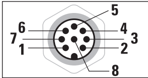
Schemazeichnung M12-Stecker
