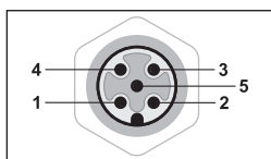
Diagrama del conector M12
