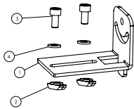
Kit di montaggio, opzionale: 240400-06
