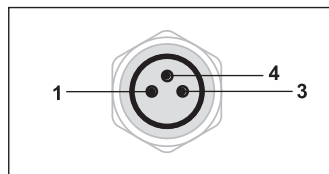
Disegno schematico connettore M8
