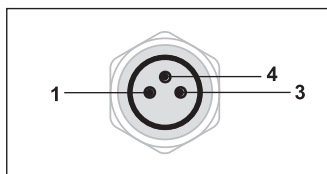
Schemazeichnung M8-Stecker
