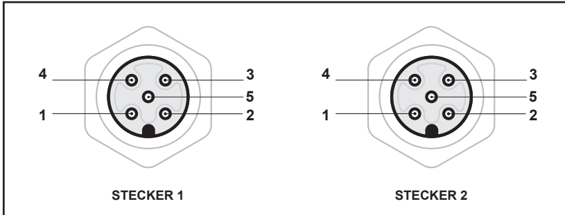
Schemazeichnung M12-Stecker
